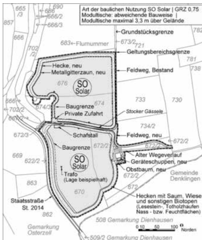
Abbildung: Lageplan, unmaßstäblich
